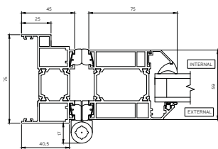
1a-1b - Hinge Jamb Detail
