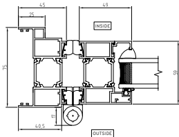
1a-1b - Hinge Jamb Detail
